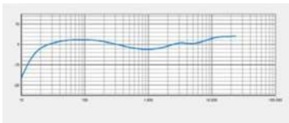
EQ Aktive version DSP-Kurve 1
